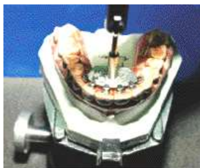
Рис. 15. Шаблонный клинок для установки брекет-систем
