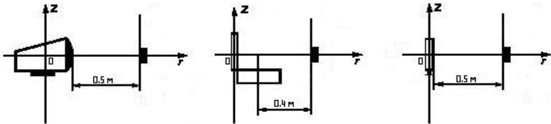
Рисунок. Расположение измерительной антенны относительно экранов дисплеев ВДТ, ЭВМ или ПЭВМ
