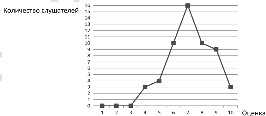
Рис. 1. Кривая распределения оценок, полученных слушателями в ходе итоговой аттестации слушателей подготовительного отделения иностранных учащихся
