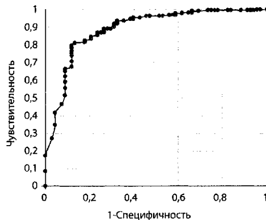
ROC-кривая прогнозной модели
