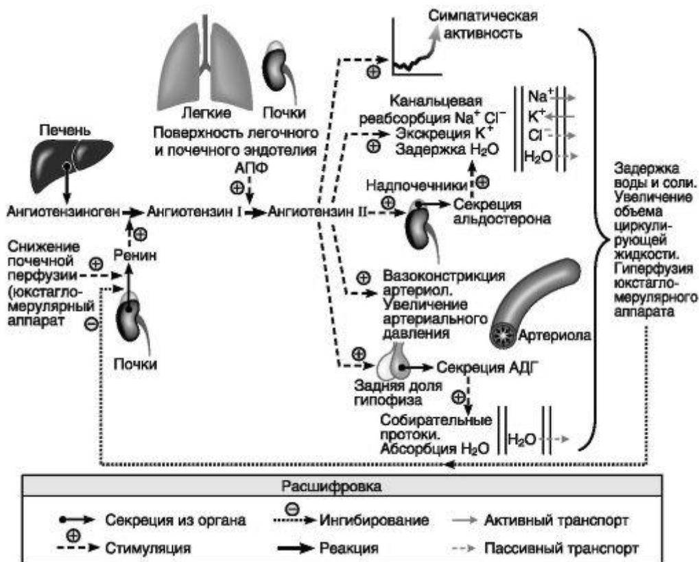
Рис. 10-1. Ренин-ангиотензин-альдостероновая система
