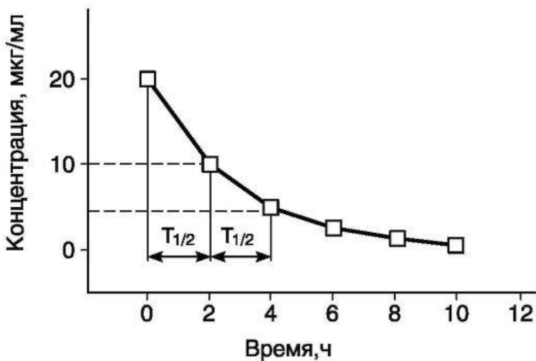
Рис. 4-4. Период полувыведения
