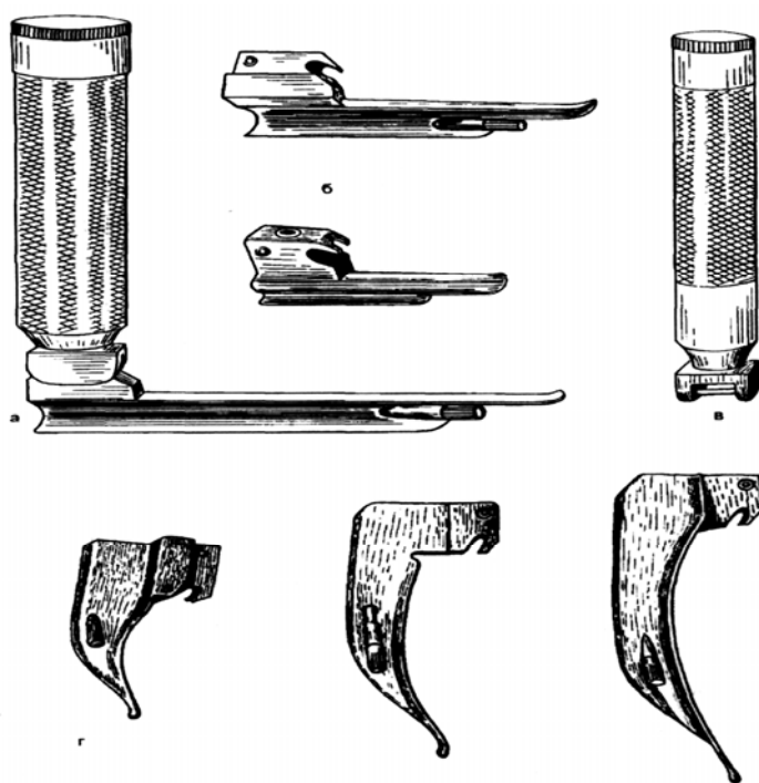
Рис. 5. Ларингоскопы. А – ларингоскоп в рабочем состоянии, б – набор прямых клинков, в – рукоятка, г – набор изогнутых клинков.
