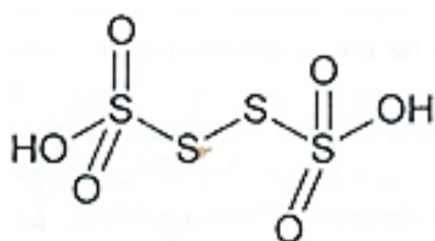
Рис. 14.3. Строение тетратионовой кислоты
