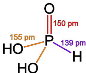
Рис. 13.4. Структура молекулы фосфористой кислоты ( H_3PO_3 )
