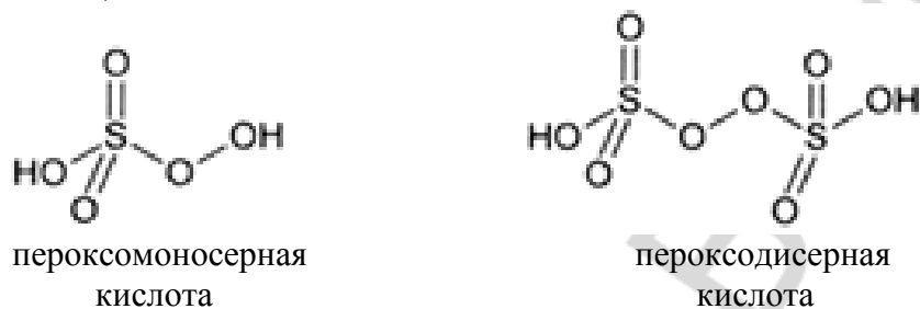
Рис. 14.5. Строение пероксокислот
