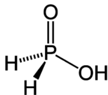
Рис. 13.3. Структура молекулы фосфорноватистой кислоты ( \text{H}_3\text{PO}_2 )
