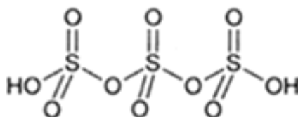
трисерная кислота
