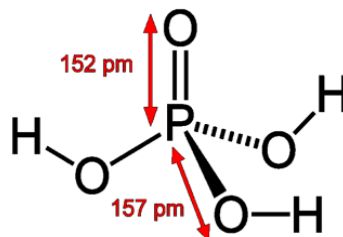
Рис. 13.6. Строение молекулы ортофосфорной кислоты
